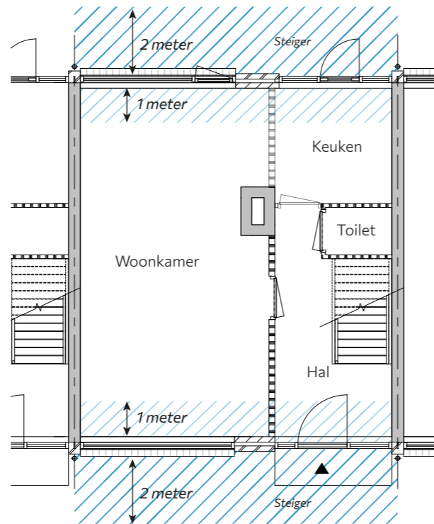
Vereiste vrije ruimte op de begane grond Dit geldt ook voor de verdieping
